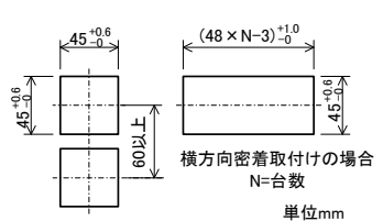
パネルカット図
