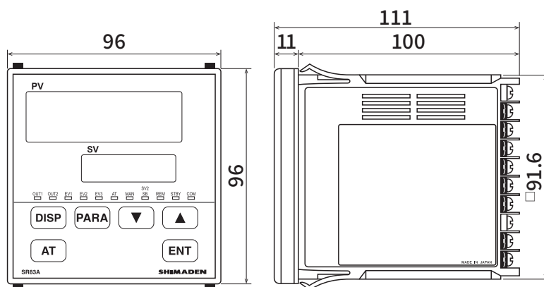
外形寸法図
