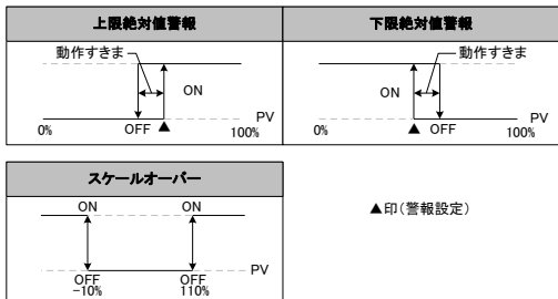
警報動作図
