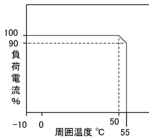
周囲温度－負荷電流特性
