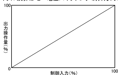
サイクル演算形ゼロ電圧スイッチング制御方式 (ZC)
