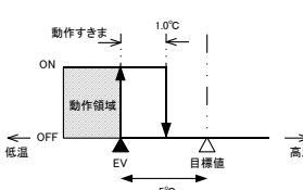
EV2 下限偏差警報動作図
