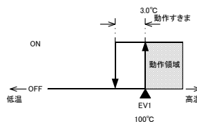
EV1 上限絶対警報動作図
