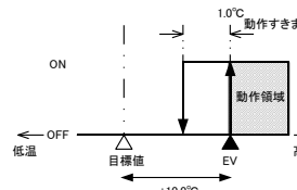
EV1 上限偏差警報動作図
