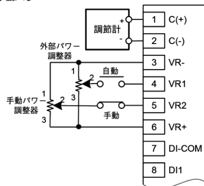
8-5-3 自動/手動切替 外部パワー調整器を使用する場合
