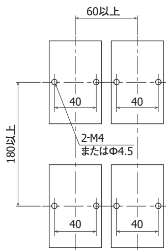
取付寸法図
