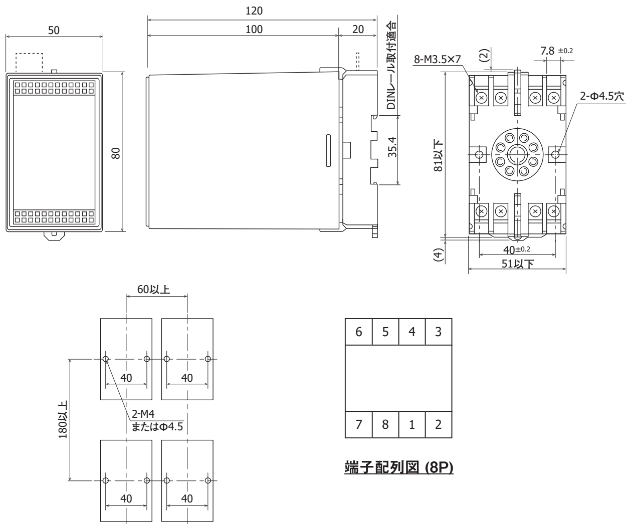
取付寸法図
