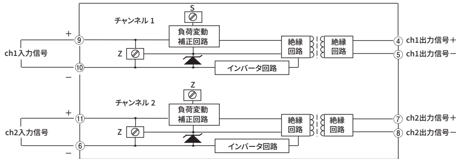
電流入力/電流出力タイプ
