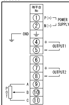
CP3737(DC24V電源)
