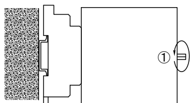
ソケットからの本体取り外し①
