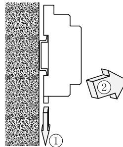
DIN レールからの取り外し
