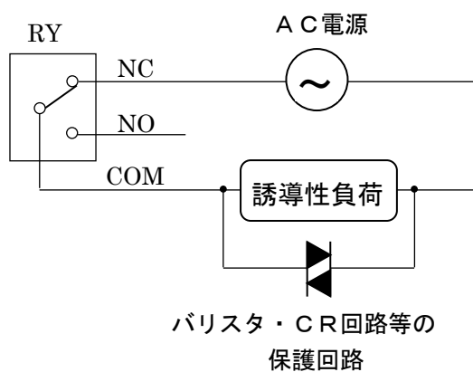
AC 電源の接続例
