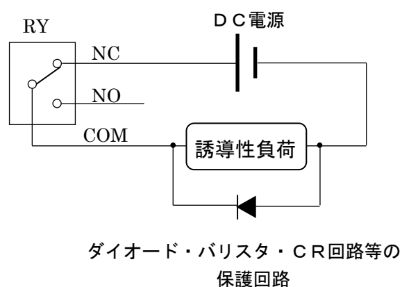
DC 電源の接続例
