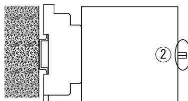
ソケットへの本体取り付け②
