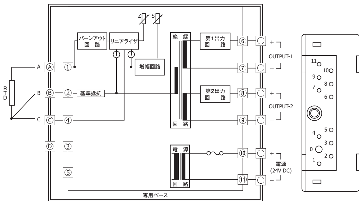
入出力ピン配置図
