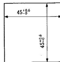
パネルカット 単位: mm
