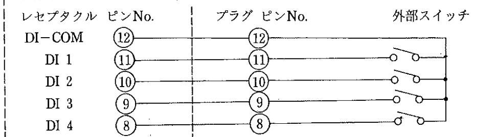
本体端子部 EXTERNAL I/O コネクター 接続図
