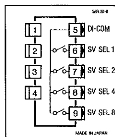
端子図
