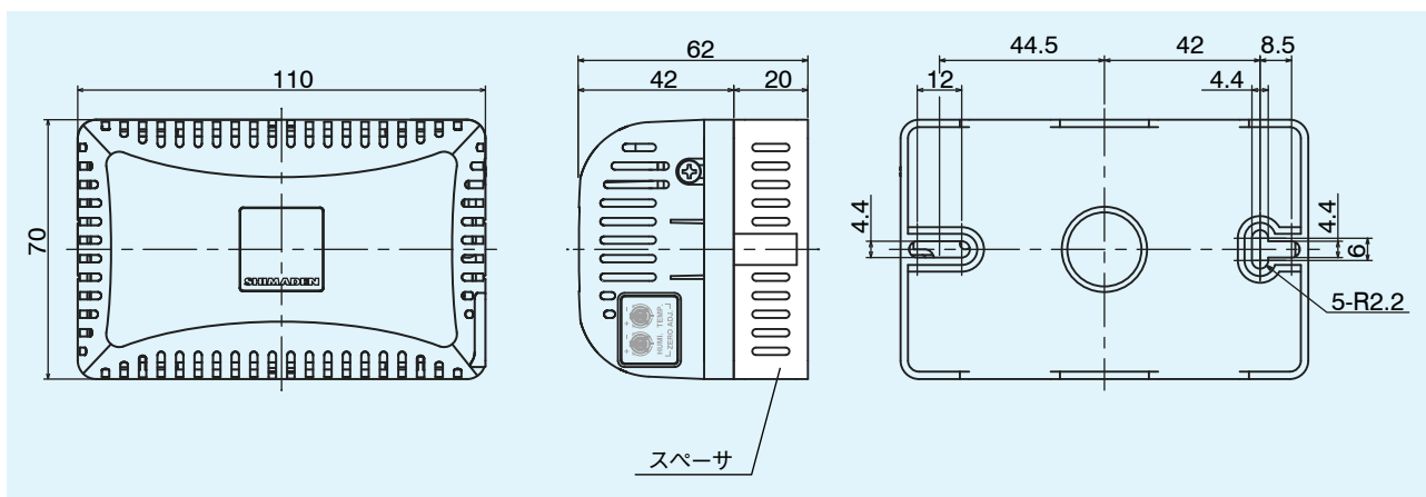
— TH71A/T71A/H71A、スペーサ付 外形寸法図 —
