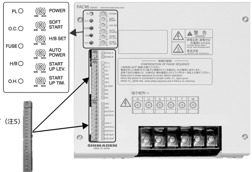
付属の端子を本体に差込む
