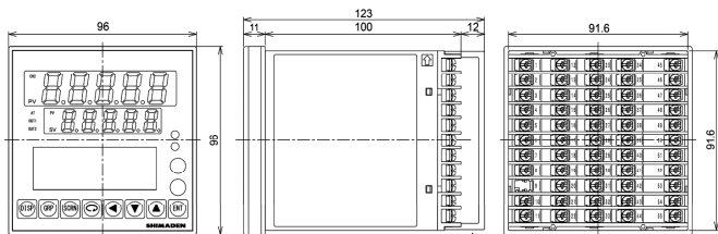
端子カバー付 単位:mm
