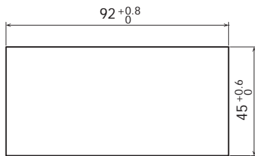
取付穴寸法
