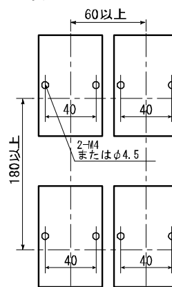
連装間隔
